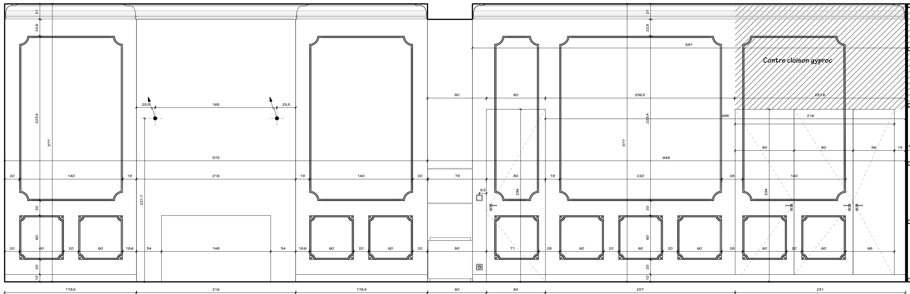
Elévation 1
