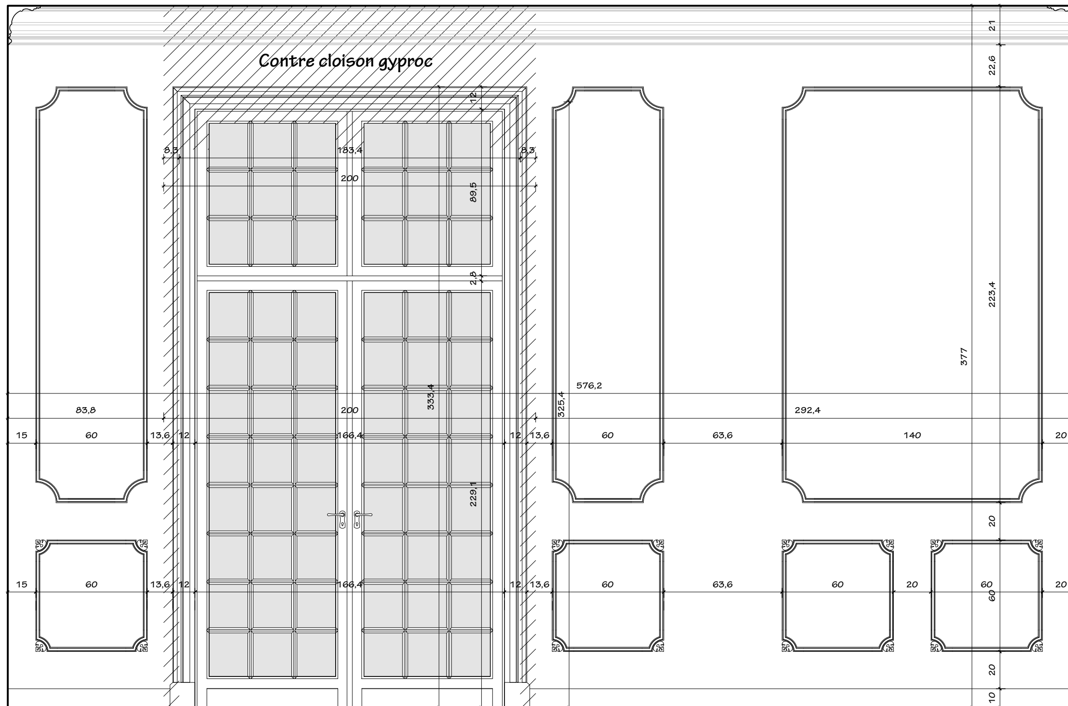
Elévation 5
