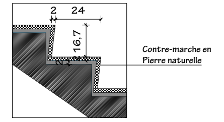
Détail Escalier Ech: 1/20
