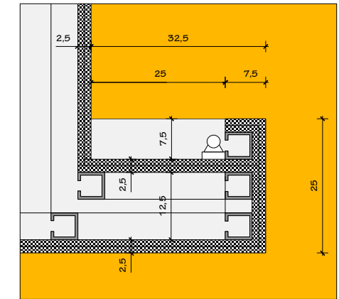
Détail gorge lumineuse Ech: 1/10
