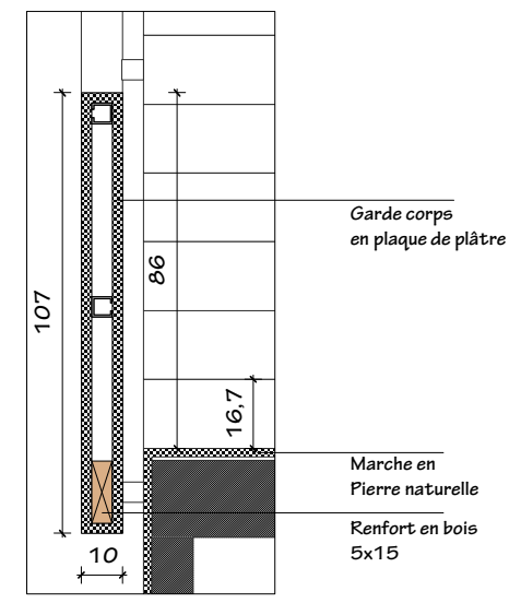
Détail garde corps Ech: 1/20
